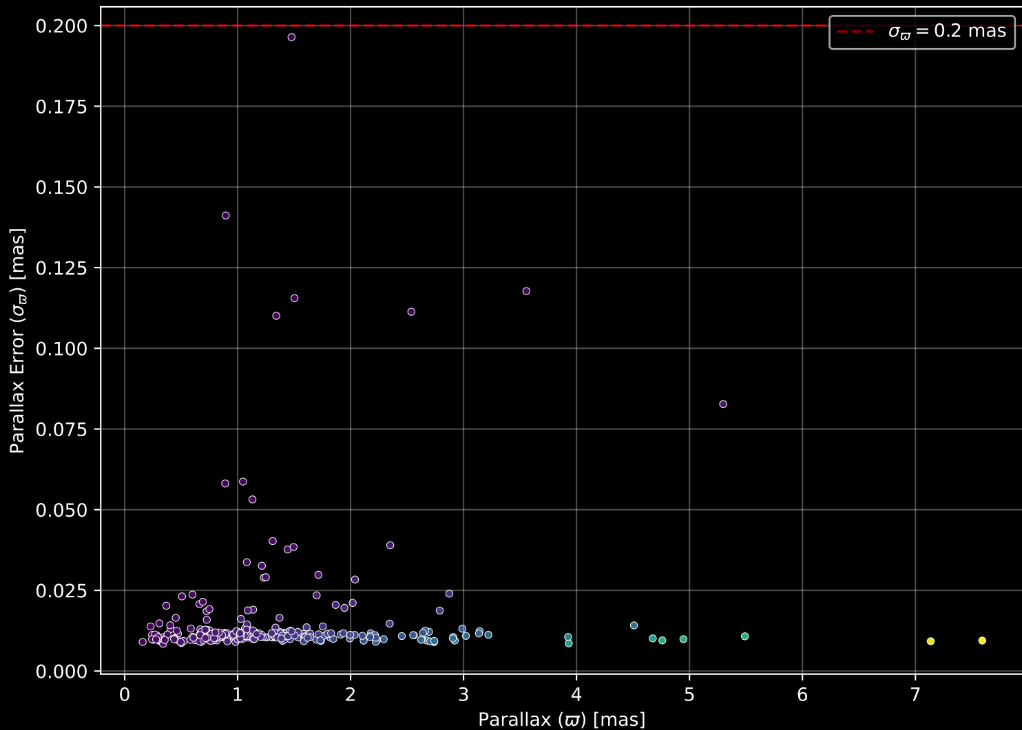
GALAH DR4 Field: [2154] Parallax Quality (n= 261)
