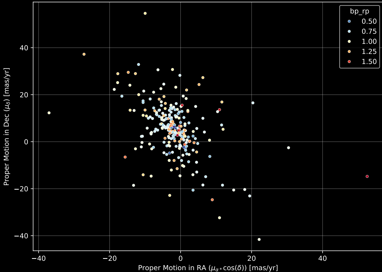
GALAH DR4 Field: [2154] Proper Motion Diagram (n= 261)
