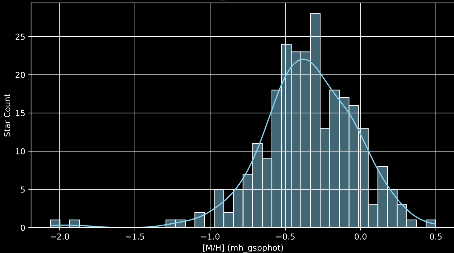
GALAH DR4 Field: [2154] [M/H] (mh_gspphot) (n= 259)
