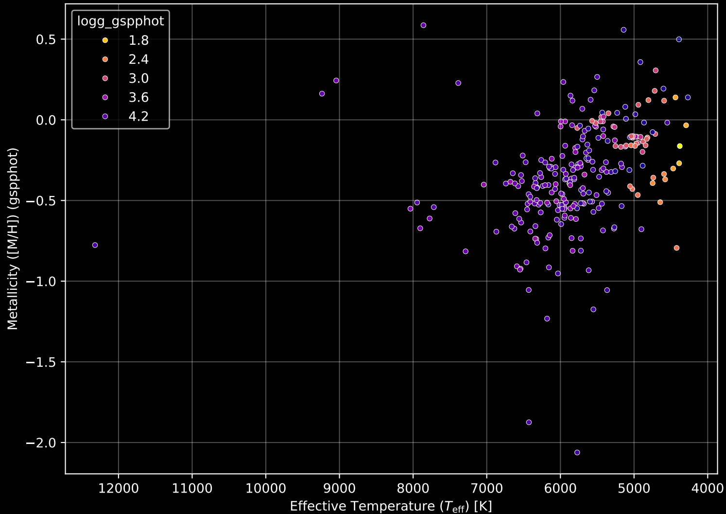
GALAH DR4 Field: [2154] Stellar Population Parameters (n= 261)
