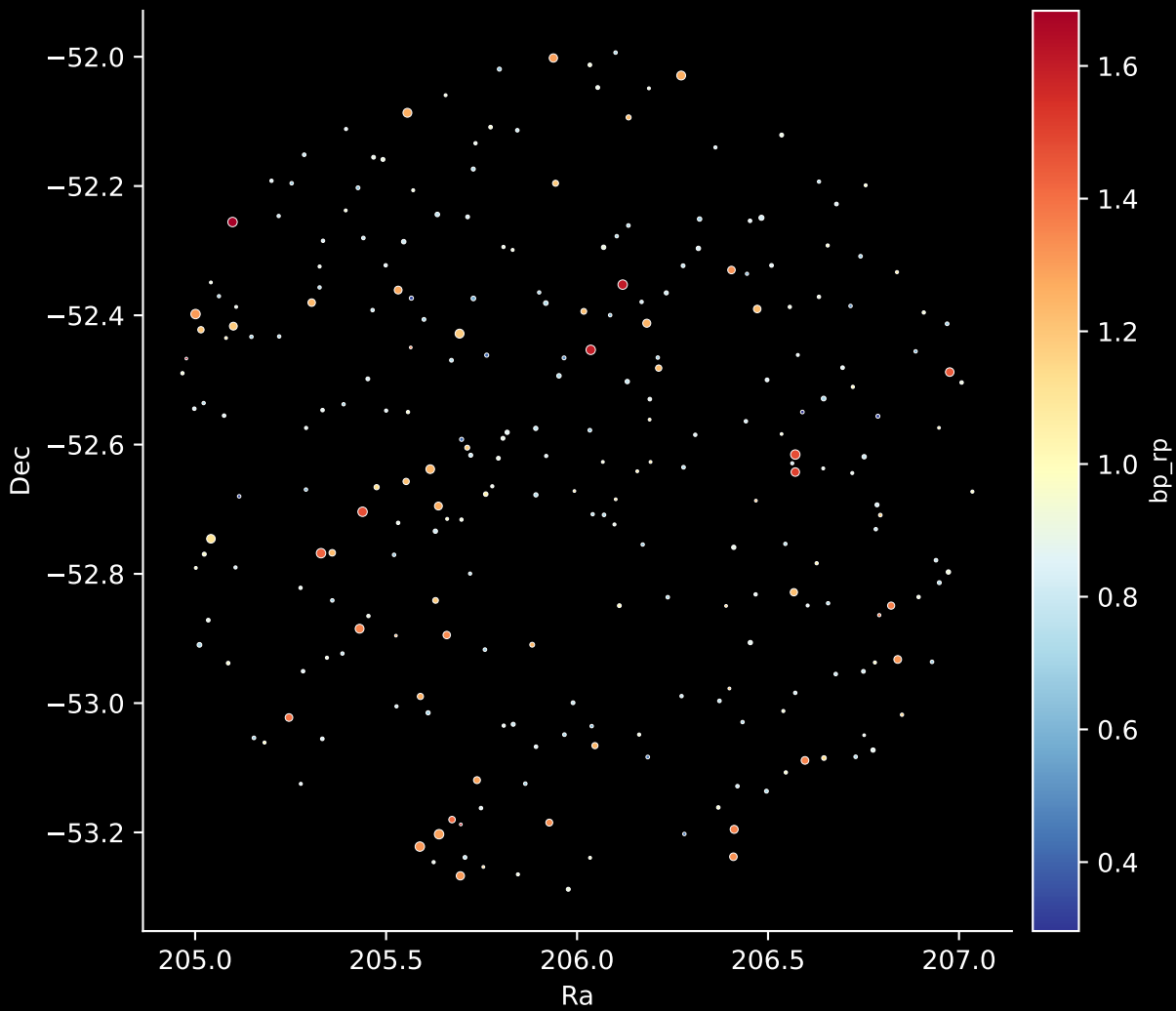
GALAH DR4 Field: [2154] Stars: 261
